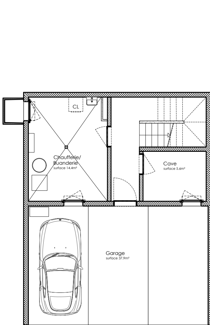
Sous-sol
