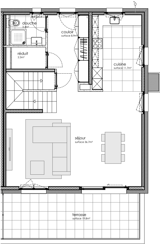
Rez-de-chaussée
