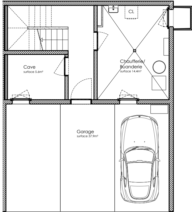
Sous-sol
